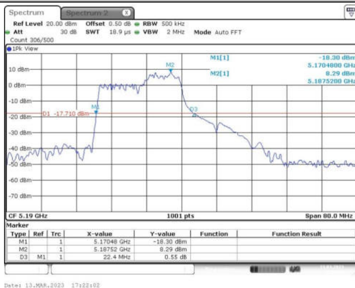
11AX40MIMO_Ant2_5190 106/54
