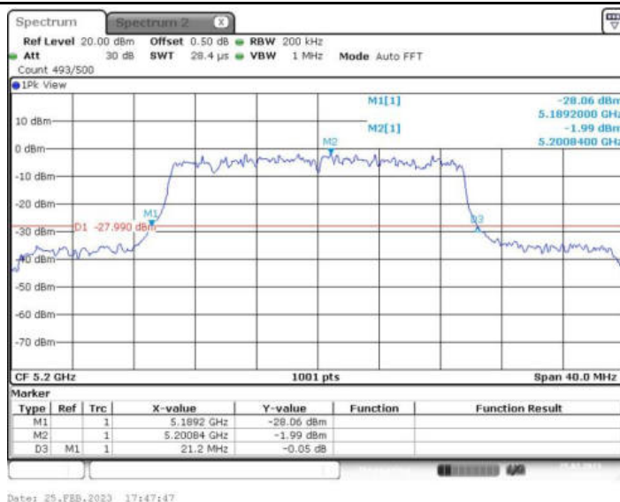
11AX20MIMO_Ant2_5200 242/61
