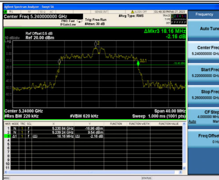
11AX20MIMO_Ant1_5240 26/4
