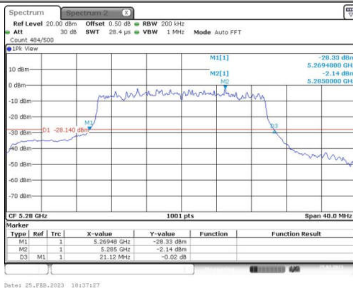
11AX20MIMO_Ant2_5280 242/61
