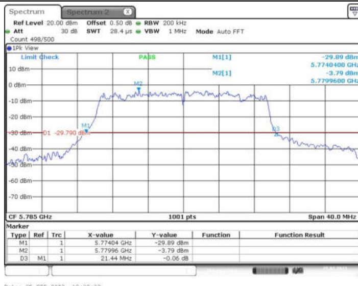
11AX20MIMO_Ant1_5785 242/61
