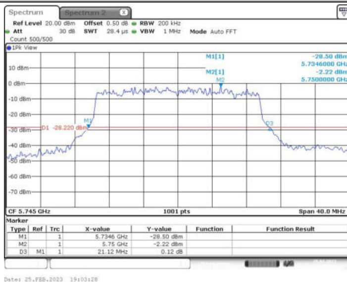
11AX20MIMO_Ant2_5745 242/61
