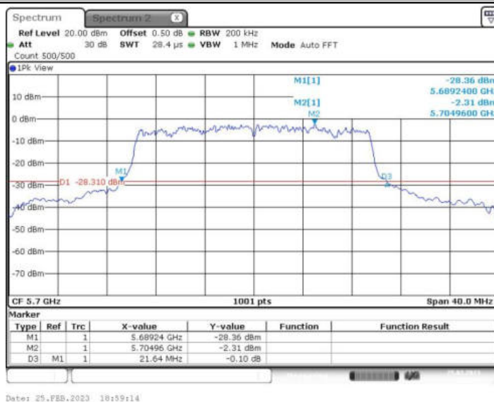
11AX20MIMO_Ant2_5700 242/61
