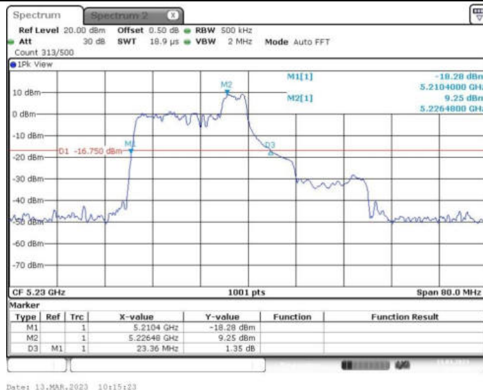
11AX40MIMO_Ant1_5230 106/54
