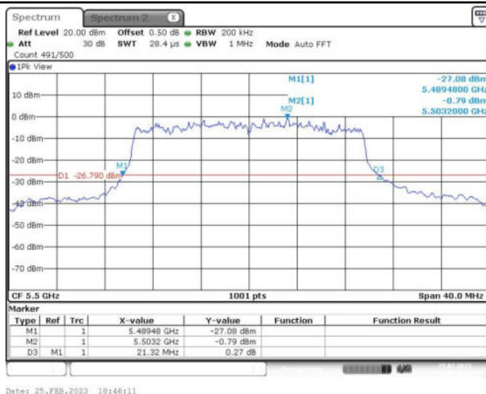
11AX20MIMO_Ant2_5500 242/61
