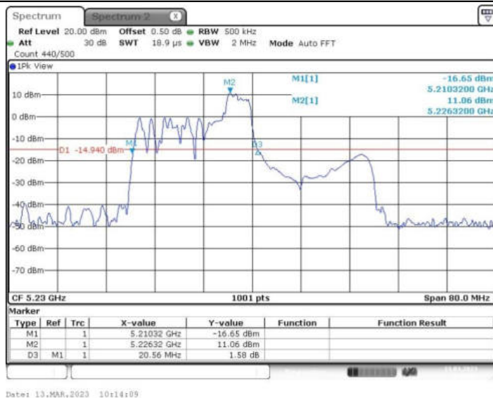
11AX40MIMO_Ant2_5230 52/40
