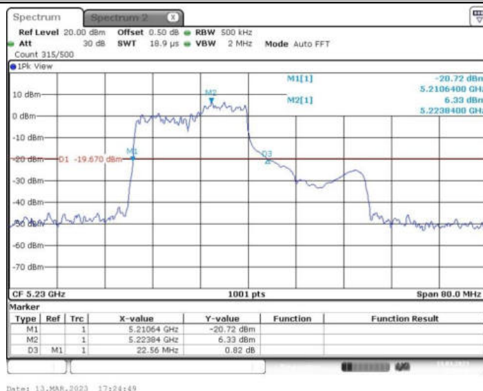
11AX40MIMO_Ant2_5230 106/54
