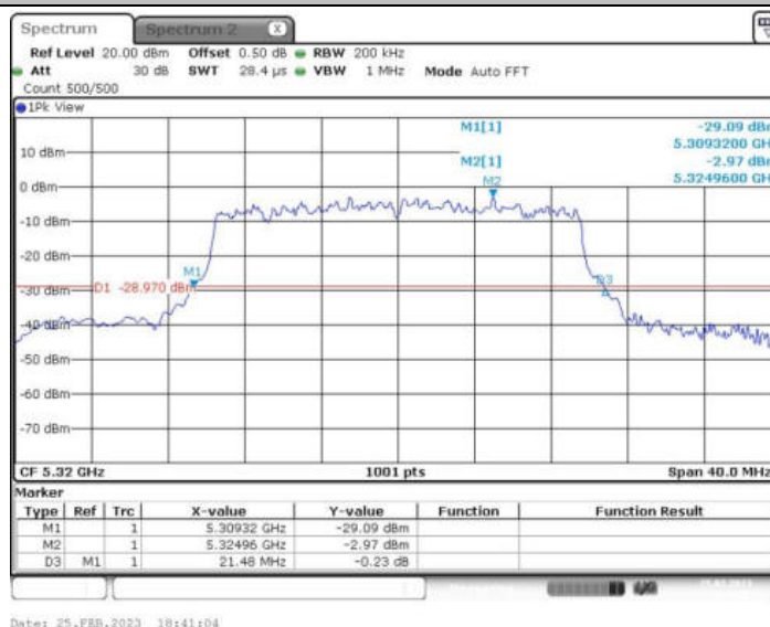
11AX20MIMO_Ant1_5320 242/61
