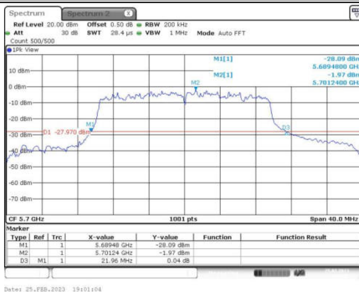
11AX20MIMO_Ant2_5700 242/61
