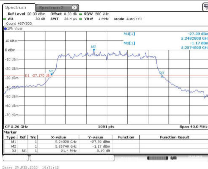
11AX20MIMO_Ant2_5260 242/61
