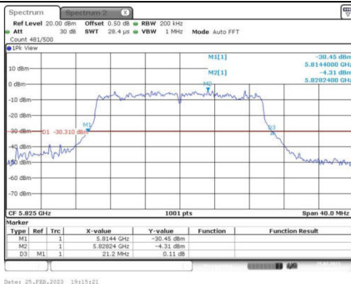
11AX20MIMO_Ant2_5825 242/61
