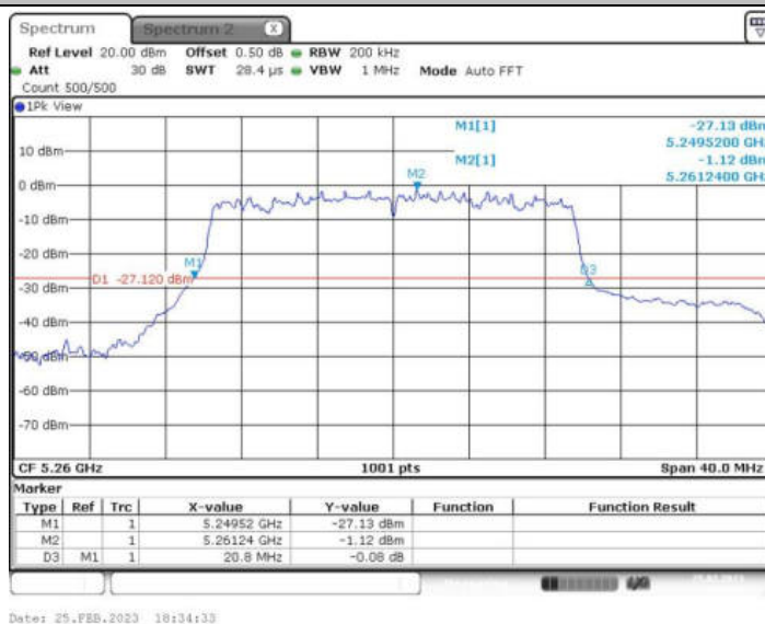
11AX20MIMO_Ant2_5260 242/61
