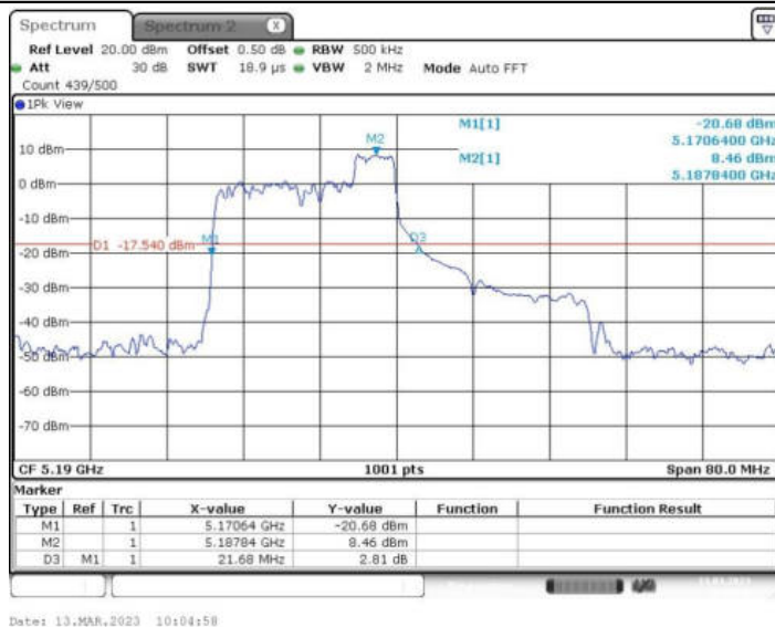
11AX40MIMO_Ant2_5190 52/40
