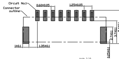
GH-nAWB PCB寸法 PCB Layout
