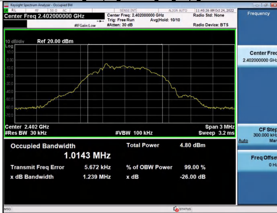
99% Occupied Bandwidth BLE 1Mbps 2402
