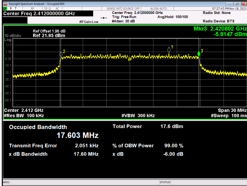
CH01: 2412MHz
