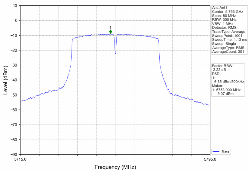
802.11n(HT40)_LCH_5755MHz_Ant1_NTNV
