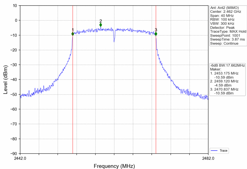
802.11n(HT20) HCH 2462MHz Ant2 (MIMO) NTV
