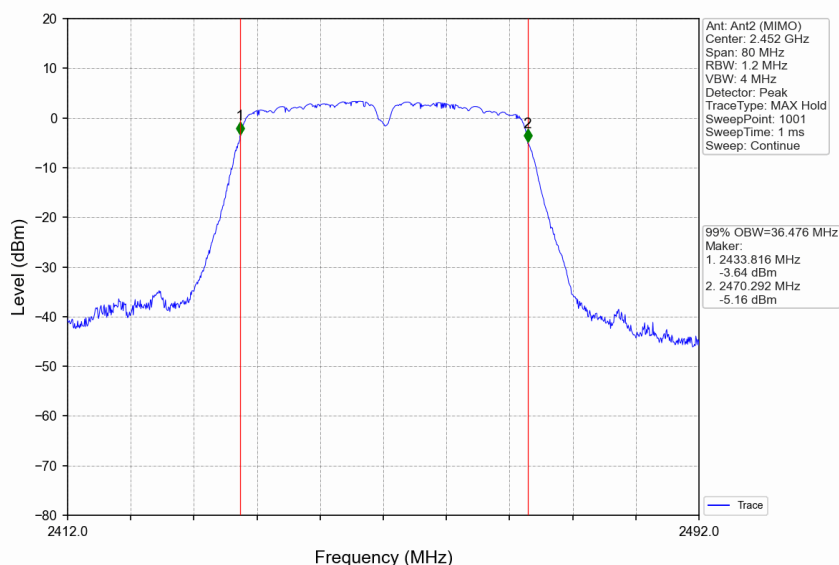
802.11n(HT40) HCH 2452MHz Ant2 (MIMO) NTV
