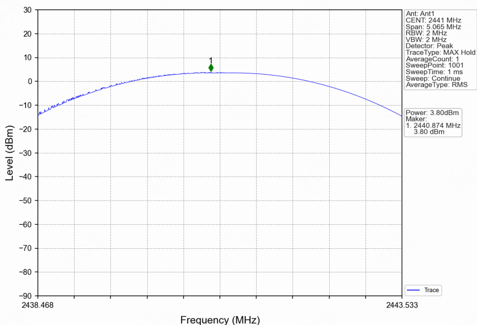
DFSK DH5 MCH 2441MHz_Ant1_NTNV
