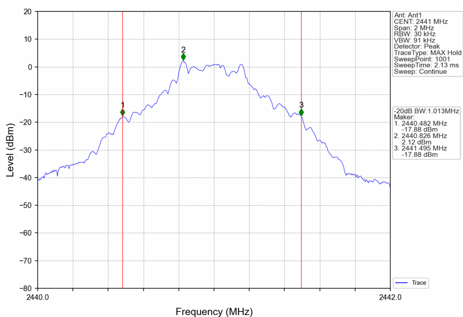
GFSK DH5 MCH 2441MHz Ant1 NTN
