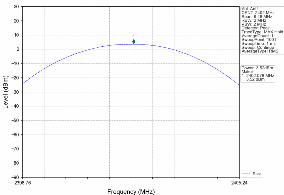
Pi/4DQPSK 2DH5 LCH 2402MHz Ant1 NTVN
