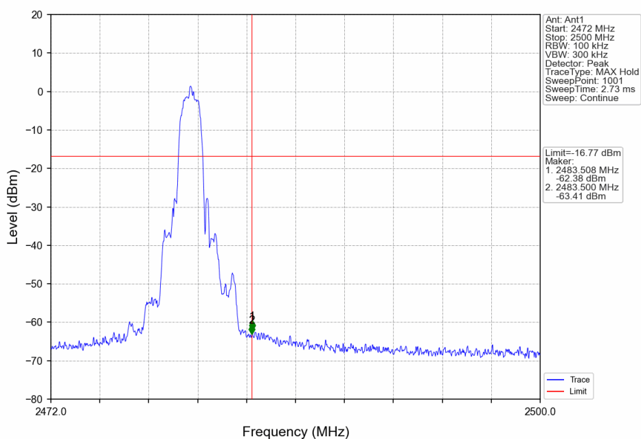
8DPSK 3DH5 HCH 2480MHz Ant1 NTN
