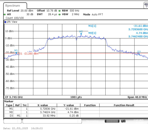
11A-Ant1-5745
