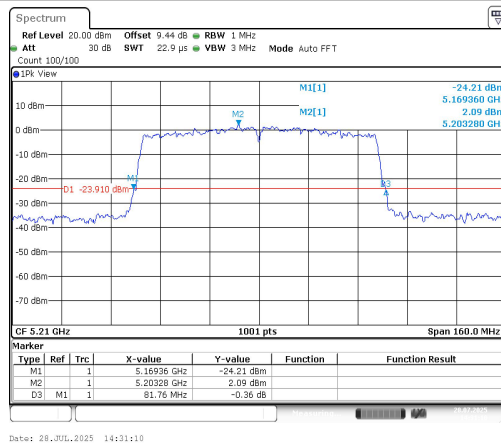
11AC80SISO-Ant1-5210
