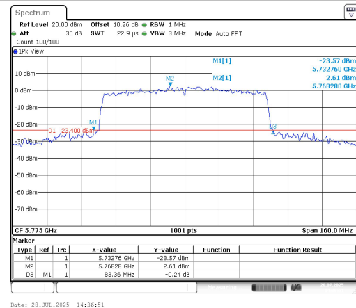
11AC80SISO-Ant1-5775
