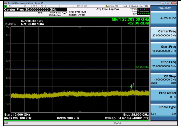
802.11n(HT20),2462MHz,Ant0,Plot 6,15000MHz~25000MHz
