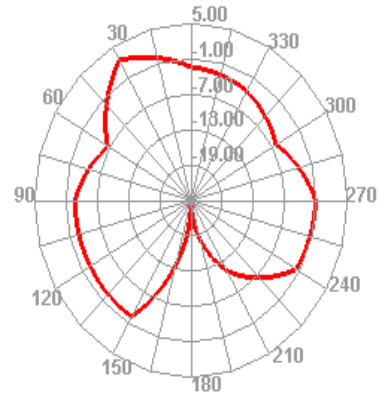
5150.000MHz H
