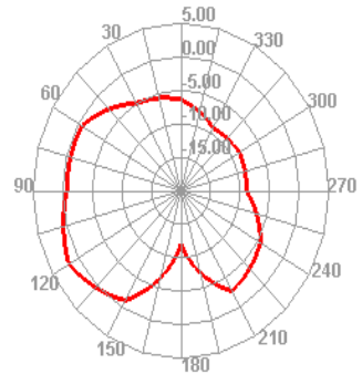
5550.000MHz E1
