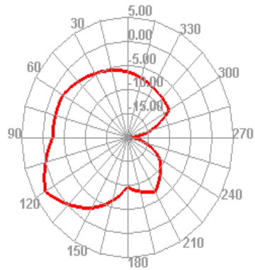
5150.000MHz E1
