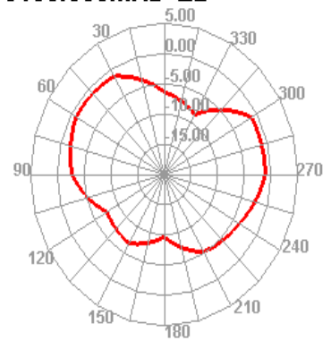
5150.000MHz E2
