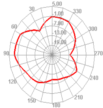
2500.000MHz H
