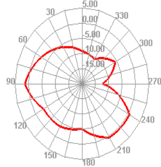
2500.000MHz E2
