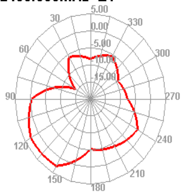
2450.000MHz E1
