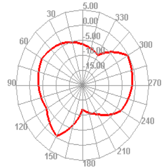
5550.000MHz E2
