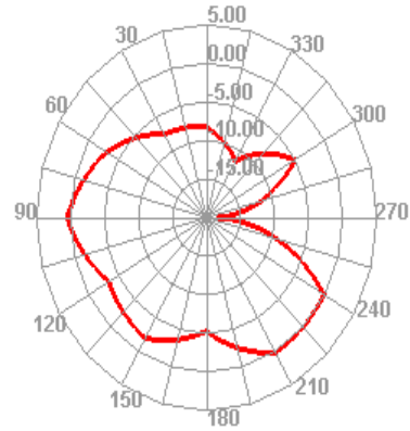
2450.000MHz E2
