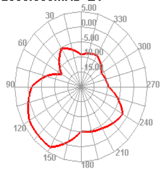
2500.000MHz E1
