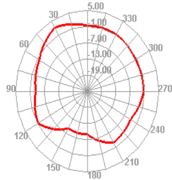
5550.000MHz H
