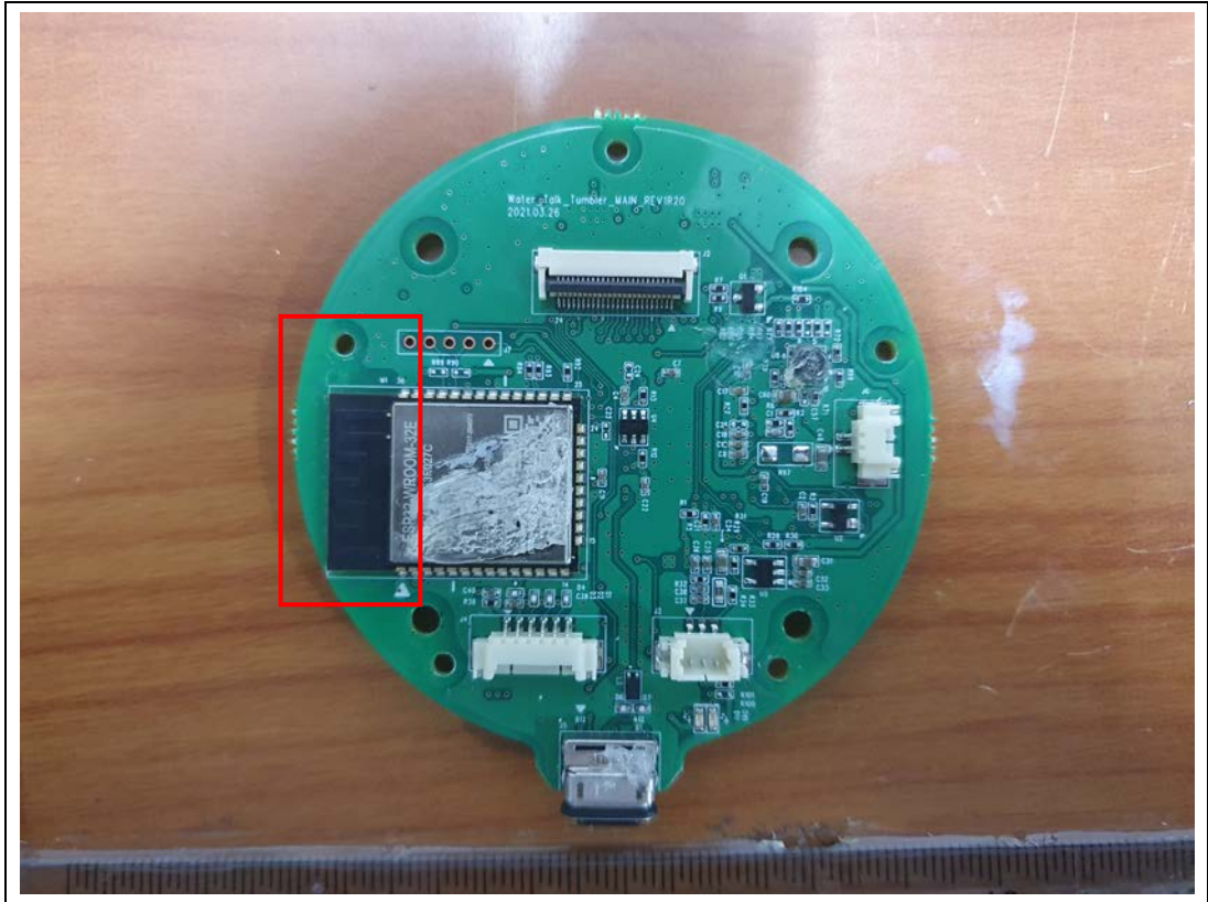
Antenna
