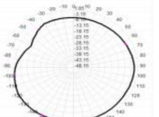
2402.0MHz Total(H), Max=-0.05dB
