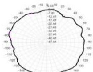
2441.0MHz Total(E2), Max=-0.09dB
