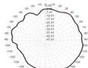
2441.0MHz Total(E1), Max=1.85dB
