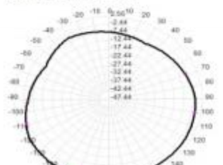
2470.0MHz Total(H), Max=2.41dB
