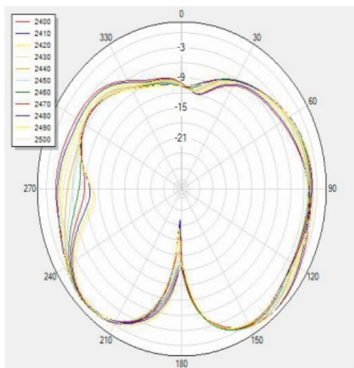
H \Theta=90
