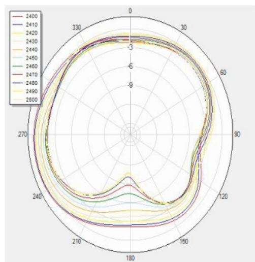
H \Theta=90
