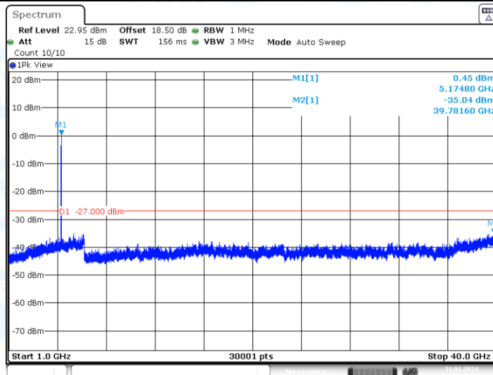
11AC20MIMO_Ant2_5180_1000~40000
