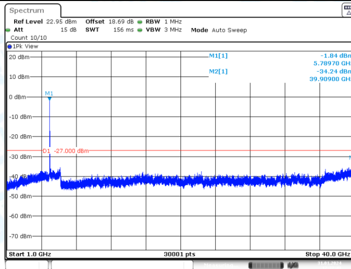
11N40MIMO_Ant1_5795_1000~40000
