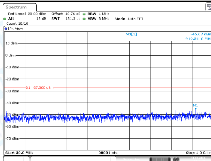
11N40MIMO_Ant2_5795_30~1000
