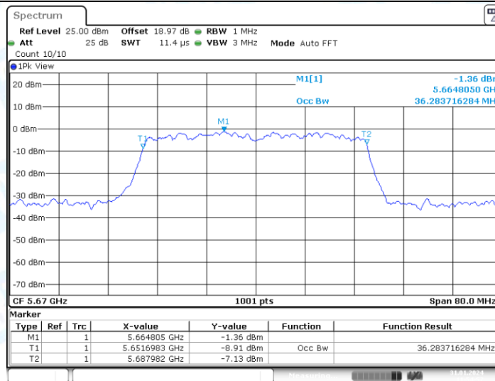
11N40MIMO_Ant2_5670
