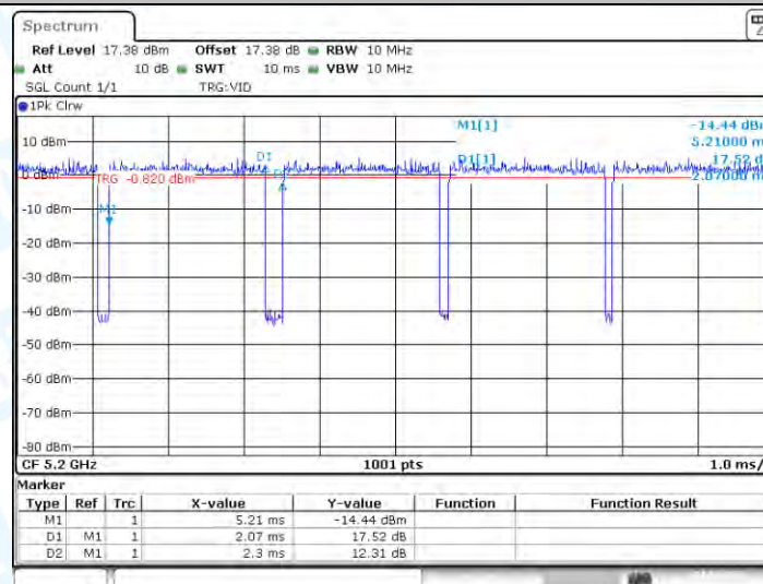
11A-CDD_Ant1_5200
