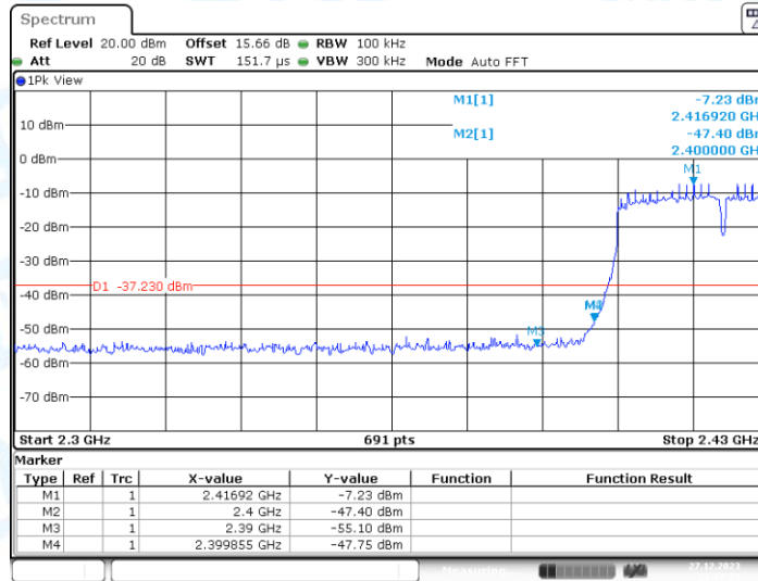
11N40MIMO_Ant2_Low_2422
