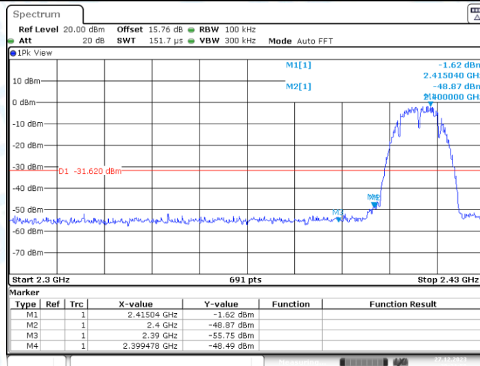
11B-CDD_Ant2_Low_2412
