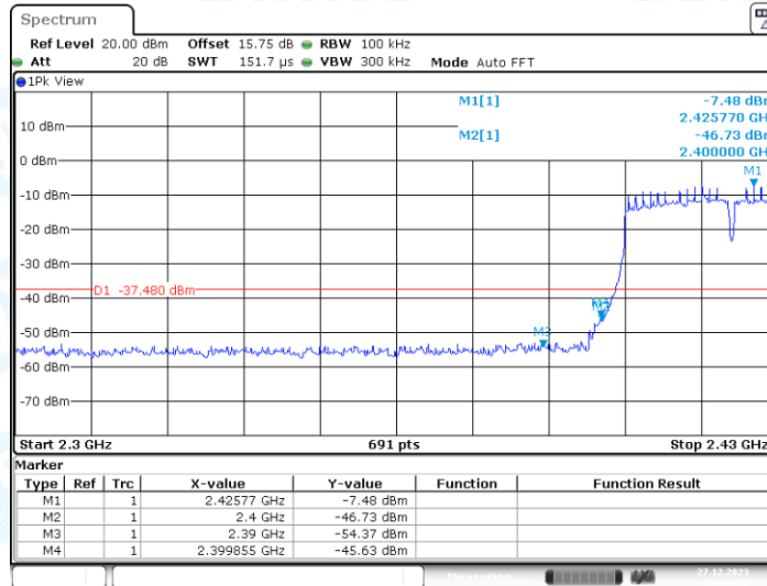
11N40MIMO_Ant2_Low_2422
