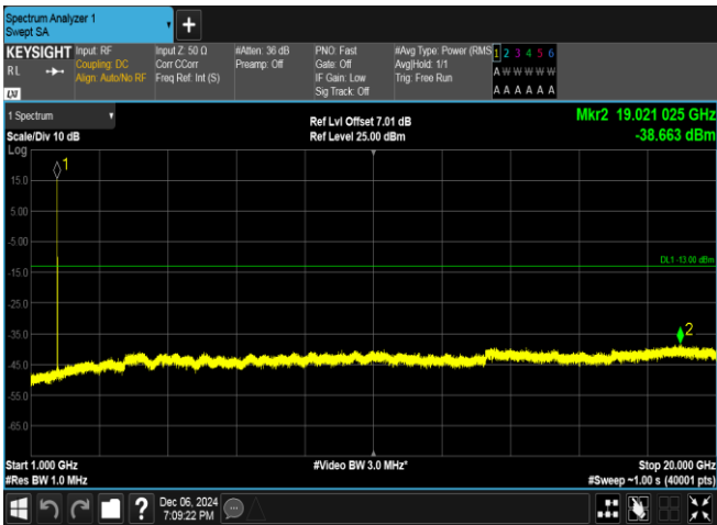
Band4-1413-4-1000~20000MHz-PASS
