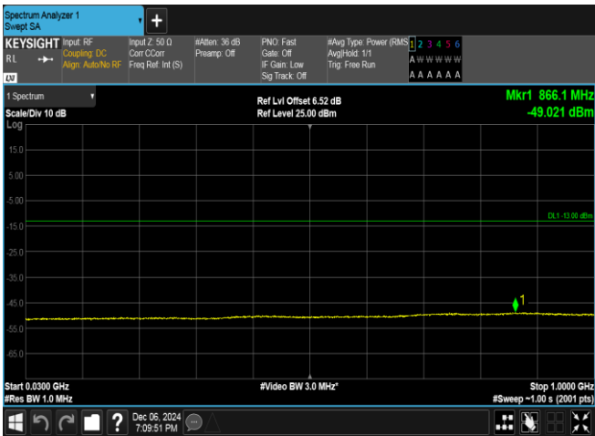
Band4-1513-4-30~1000MHz-PASS
