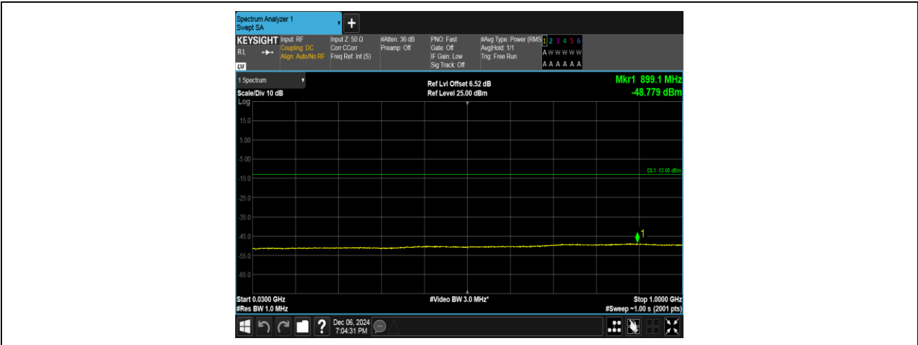
Band4-1312-2-30~1000MHz-PASS
