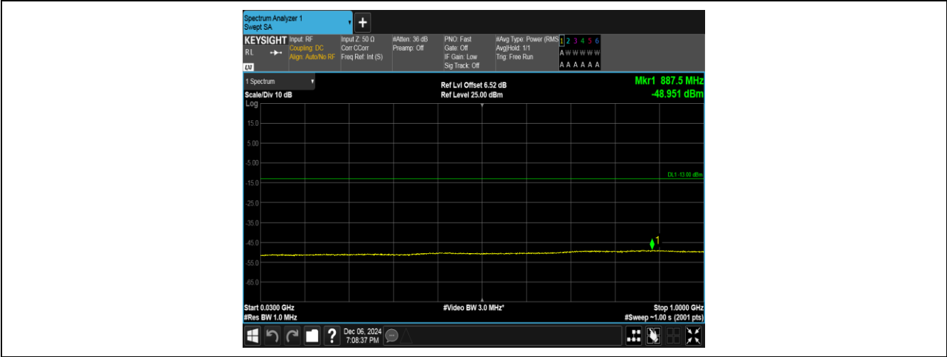
Band4-1312-4-30~1000MHz-PASS
