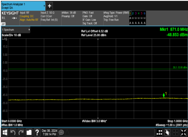
Band4-1413-4-30~1000MHz-PASS
