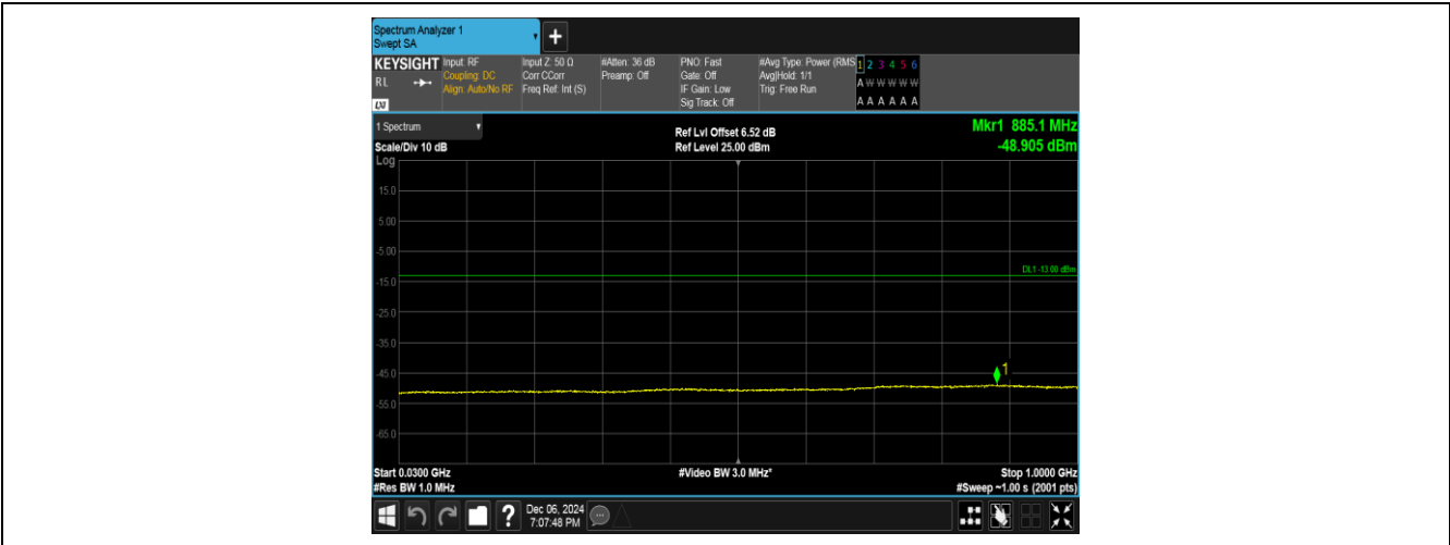
Band4-1513-3-30~1000MHz-PASS
