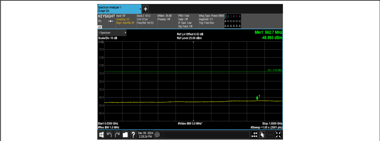
Band2-9400-1-30~1000MHz-PASS
