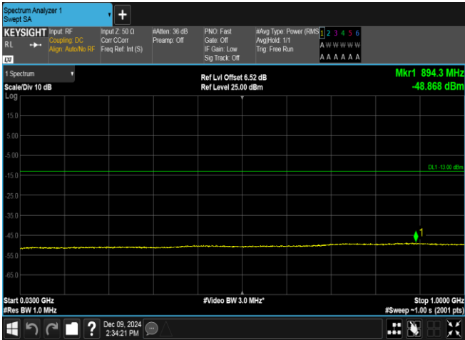
Band2-9400-3-30~1000MHz-PASS
