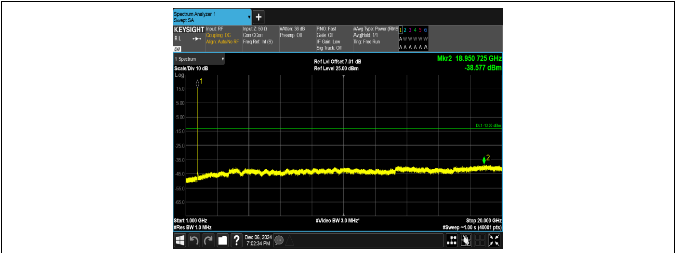
Band4-1312-1-1000~20000MHz-PASS
