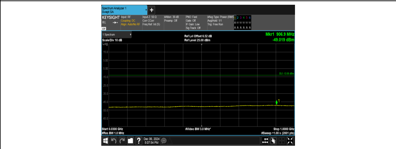
Band2-9538-2-30~1000MHz-PASS
