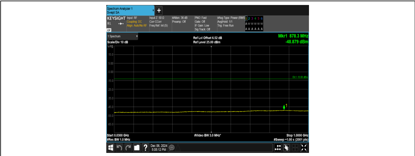
Band2-9400-1-30~1000MHz-PASS
