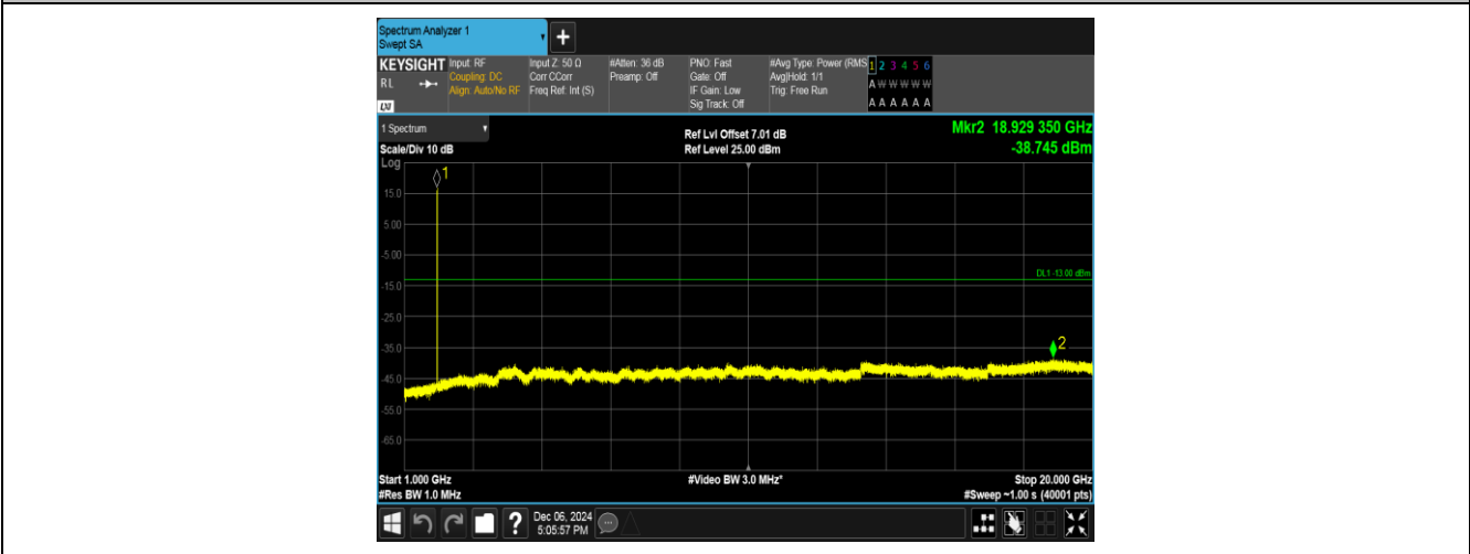
Band2-9538-1-1000~20000MHz-PASS
