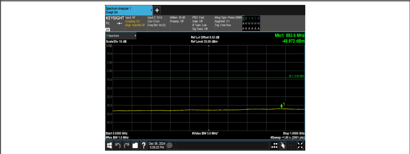
Band2-9400-3-30~1000MHz-PASS
