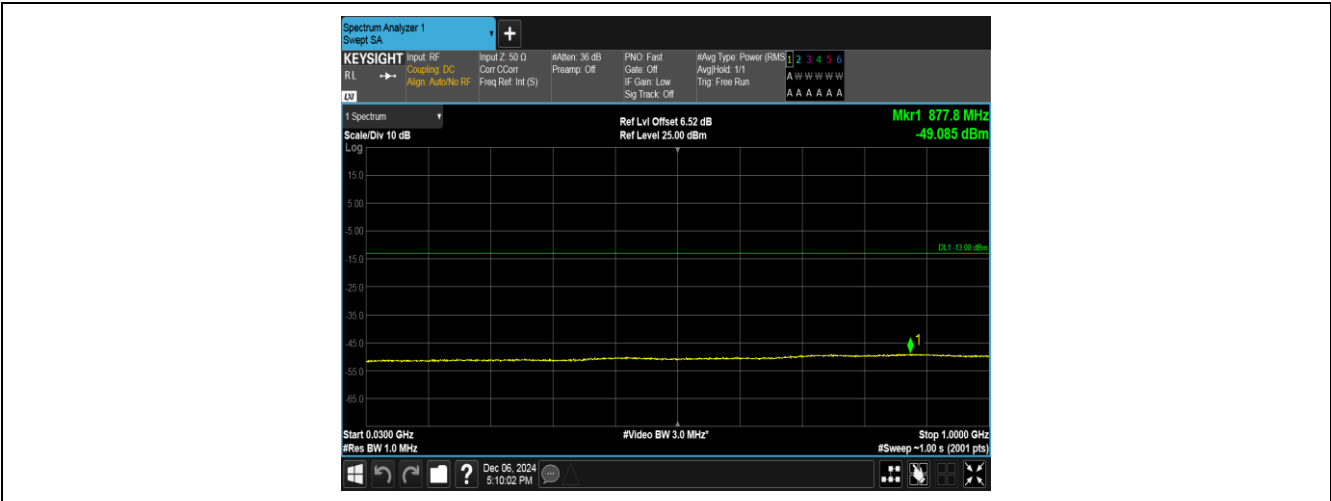
Band2-9538-3-30~1000MHz-PASS
