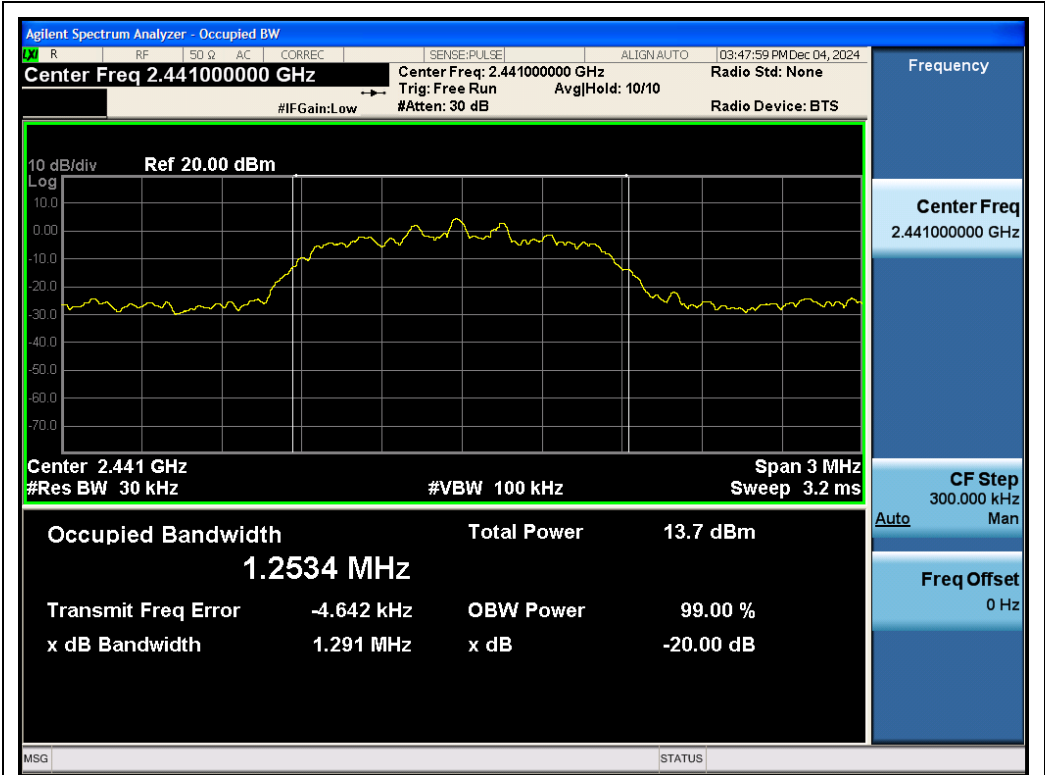
Test_Graph_EDR_ANT1_2441_2Mbps_OBW
