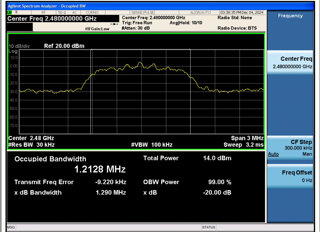
Test_Graph_EDR_ANT1_2480_2Mbps_OBW
