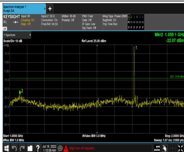
Band66-10MHz-QPSK-132022-1RB#0-Range2:1000~2000MHz
