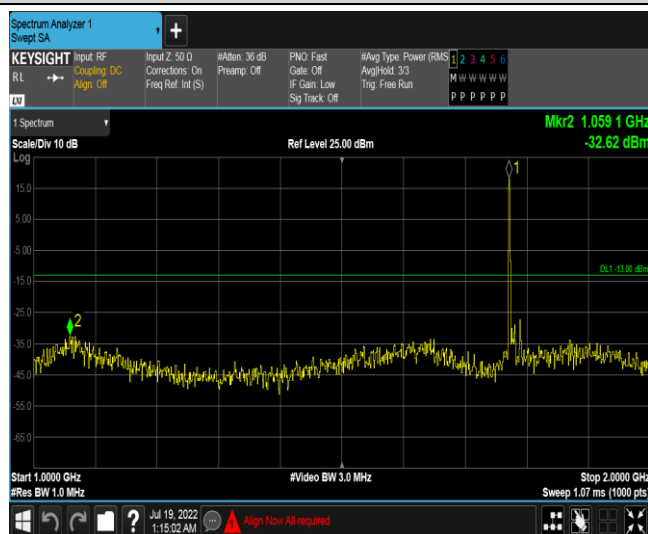
Band66-10MHz-QPSK-132622-1RB#0-Range2:1000~2000MHz
