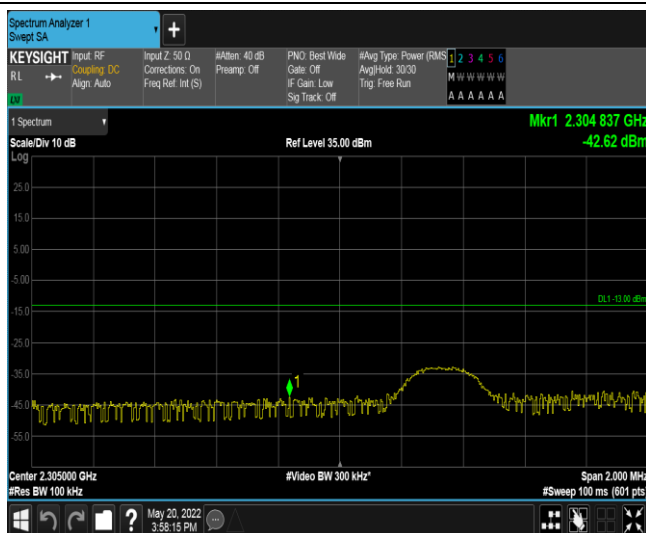
Band40-5MHz-QPSK-38725-25RB#0
