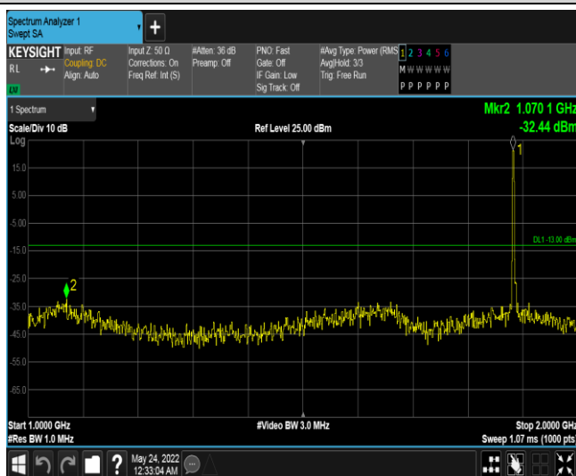
Band25-3MHz-QPSK-26365-1RB#0-Range2:1000~2000MHz
