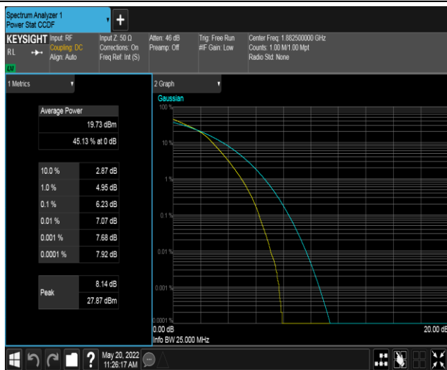
Band25-20MHz-16QAM-26365-100RB#0
