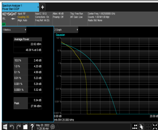
Band25-20MHz-QPSK-26365-100RB#0
