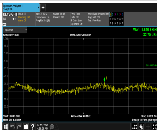
Band19-5MHz-QPSK-24075-1RB#0-Range2:1000~2000MHz
