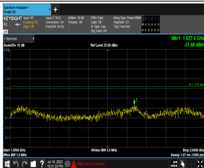
Band18-10MHz-QPSK-23900-1RB#0-Range2:1000~2000MHz
