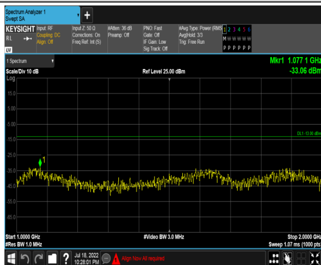
Band18-5MHz-QPSK-23925-1RB#0-Range2:1000~2000MHz
