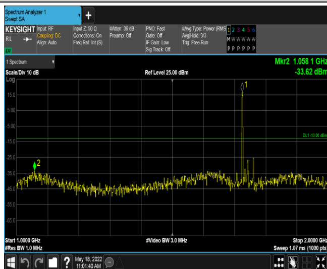
Band4-20MHz-QPSK-20175-1RB#0-Range2:1000~2000MHz
