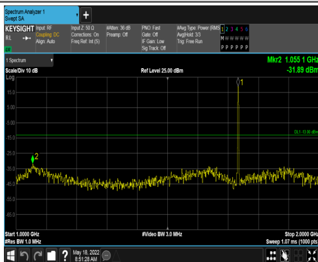
Band4-1.4MHz-QPSK-20175-1RB#0-Range2:1000~2000MHz
