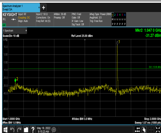
Band4-3MHz-QPSK-19965-1RB#0-Range2:1000~2000MHz
