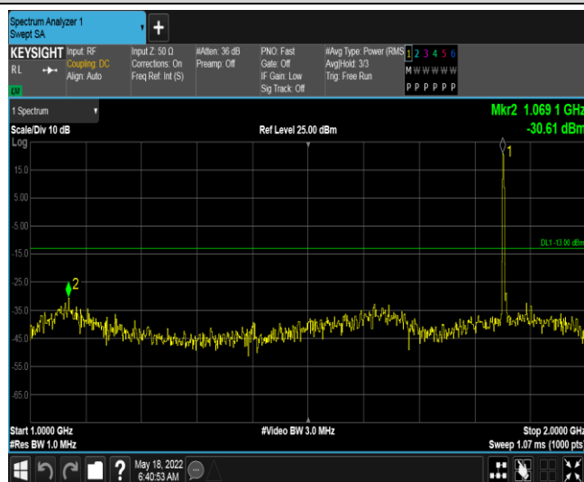
Band2-3MHz-QPSK-18615-1RB#0-Range2:1000~2000MHz
