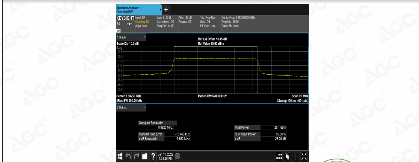
Band25-10MHz-QPSK-26365-50RB#0
