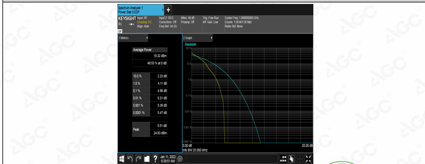
Band2-20MHz-QPSK-19100-1RB#0
