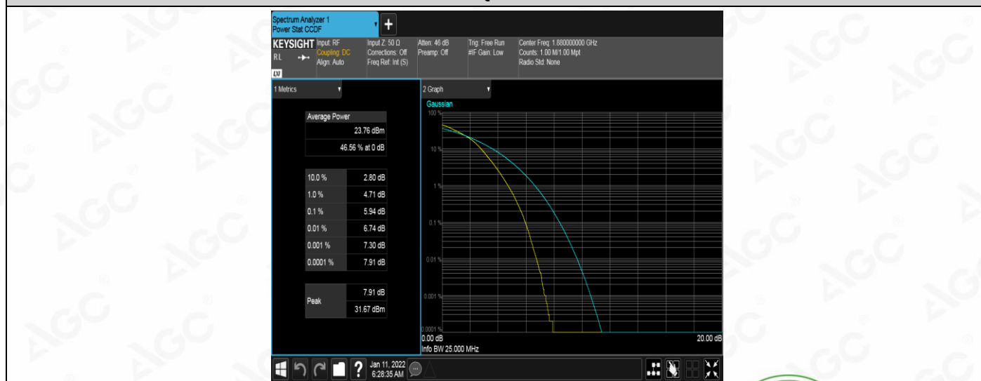
Band2-20MHz-16QAM-18900-100RB#0
