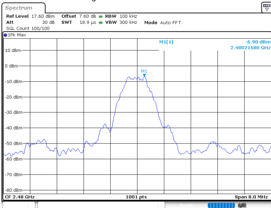
Band Edge NVNT BLE 2480MHz Ant1 Emission
