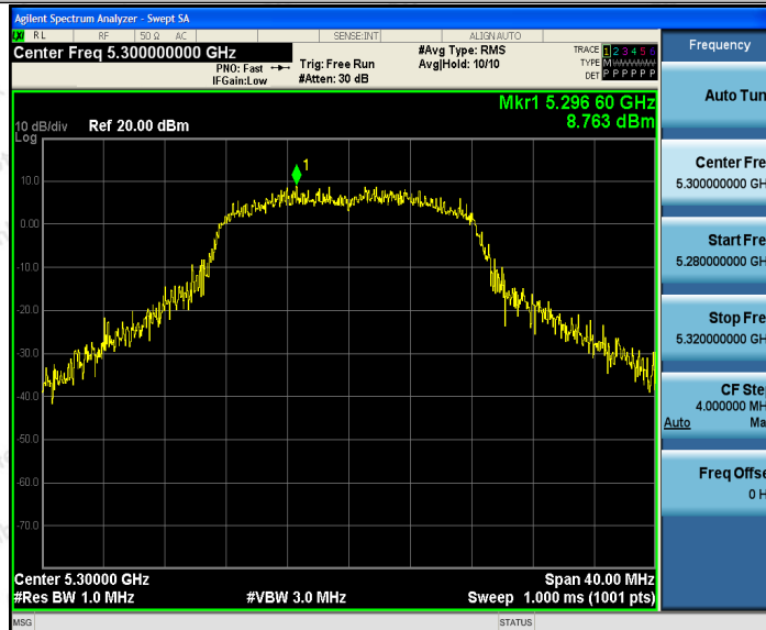
11A_Ant2_5300
