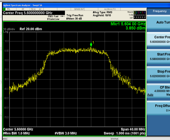
11N20SISO_Ant2_5600
