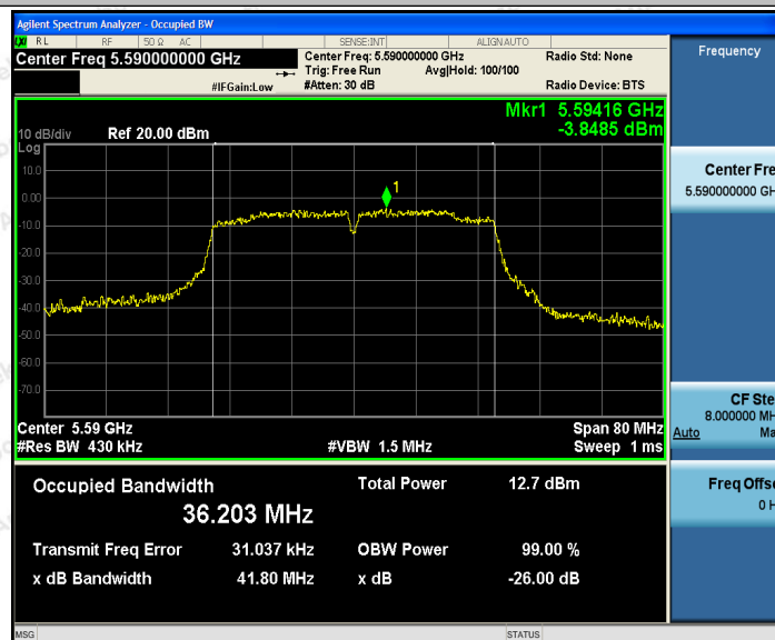
11N40SISO_Ant2_5590
