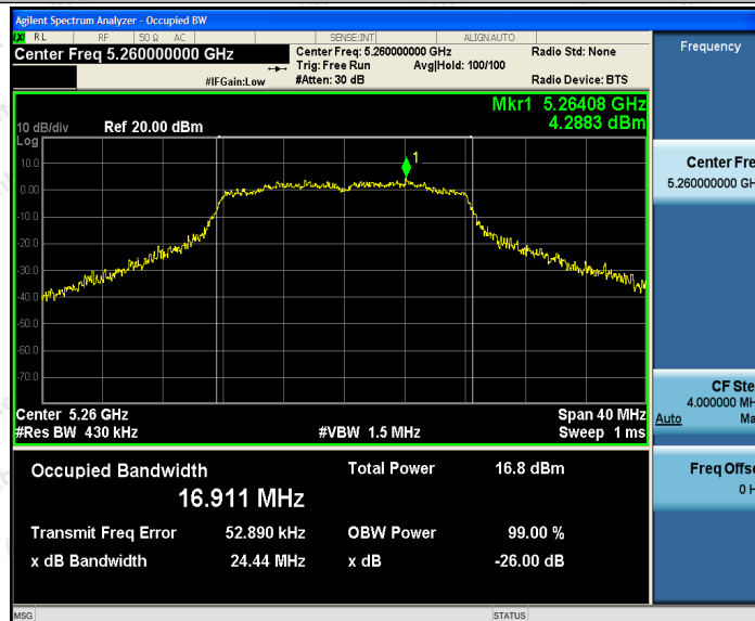
11A_Ant2_5260
