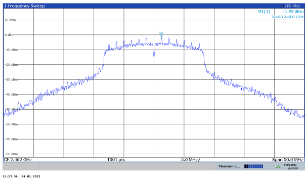
2462 MHz
