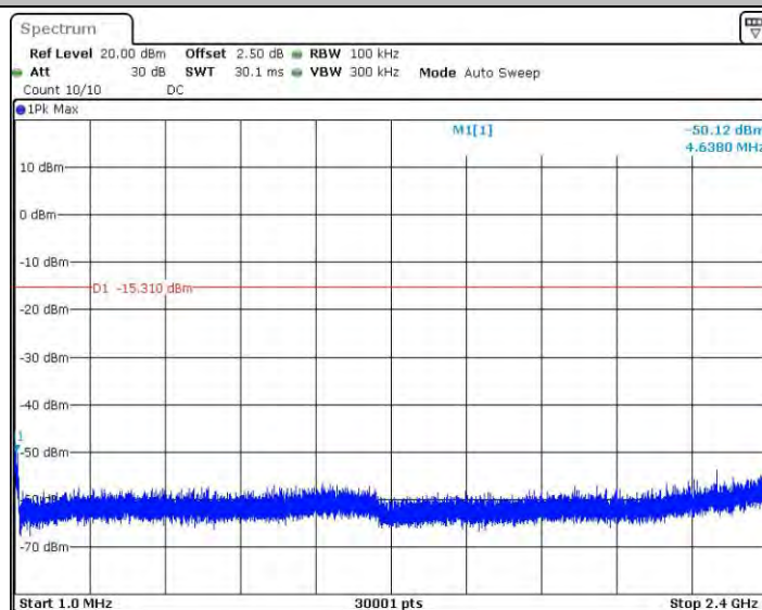
11G_Ant2_2462_1~2400
