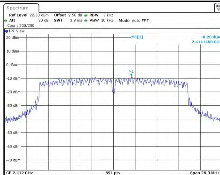
11N20_Ant2_2412
