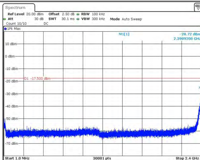
11N40_Ant2_2437_1~2400
