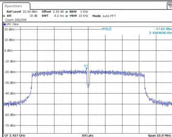
11N40_Ant2_2437
