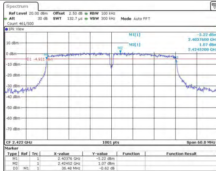
11N40_Ant1_2422
