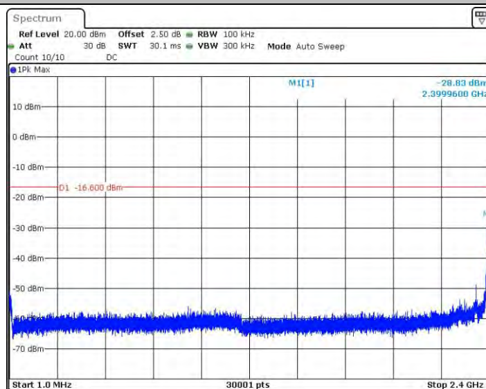
11G_Ant1_2412_1~2400
