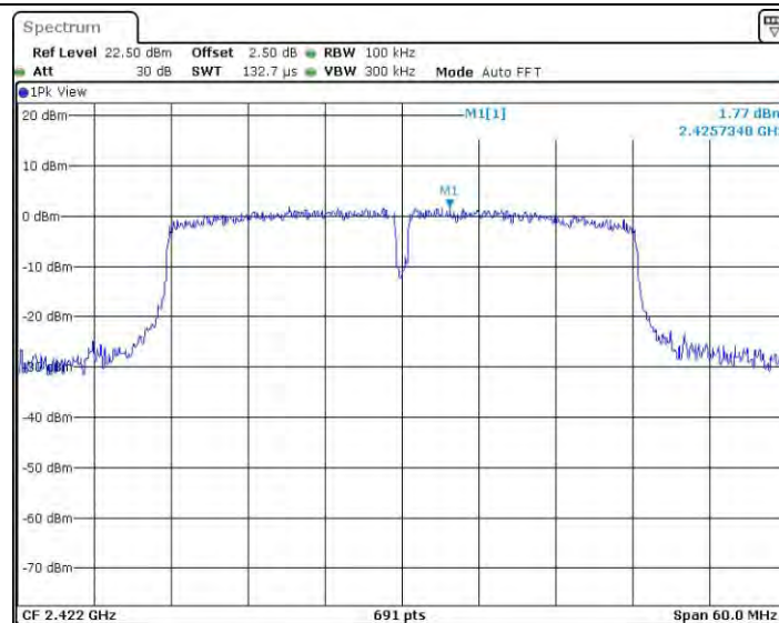
11N40_Ant2_2422_0~Reference
