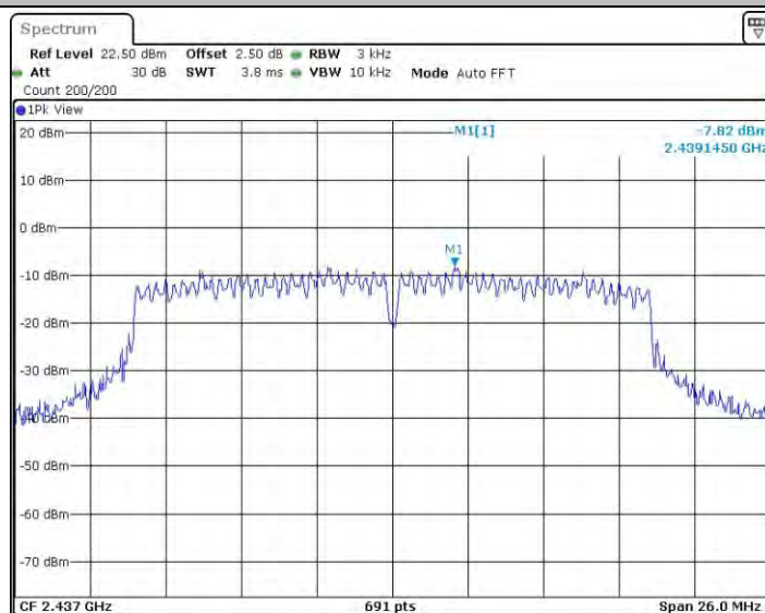
11N20_Ant2_2437
