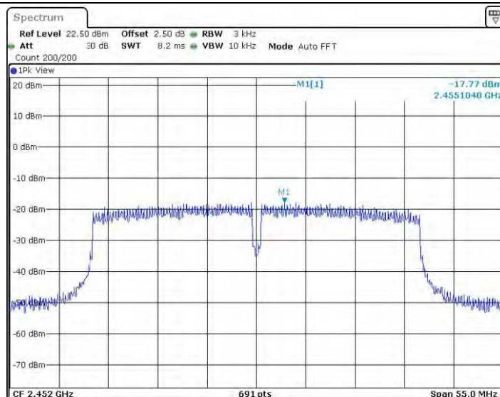
11N40_Ant2_2452
