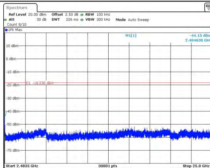
11N40_Ant2_2422_2483.5~25000
