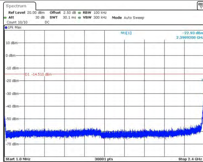
11N20_Ant2_2412_1~2400
