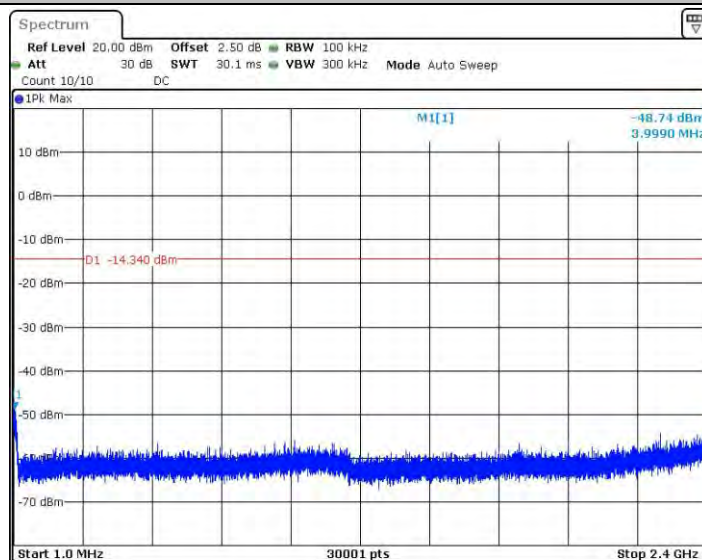
11N20_Ant2_2462_1~2400
