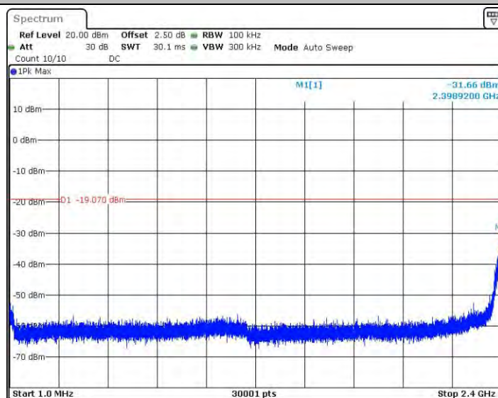
11N40_Ant1_2422_1~2400
