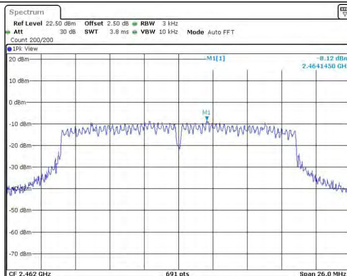
11N20_Ant2_2462
