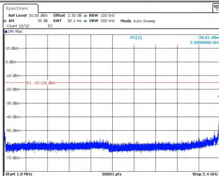
11N20_Ant1_2412_1~2400
