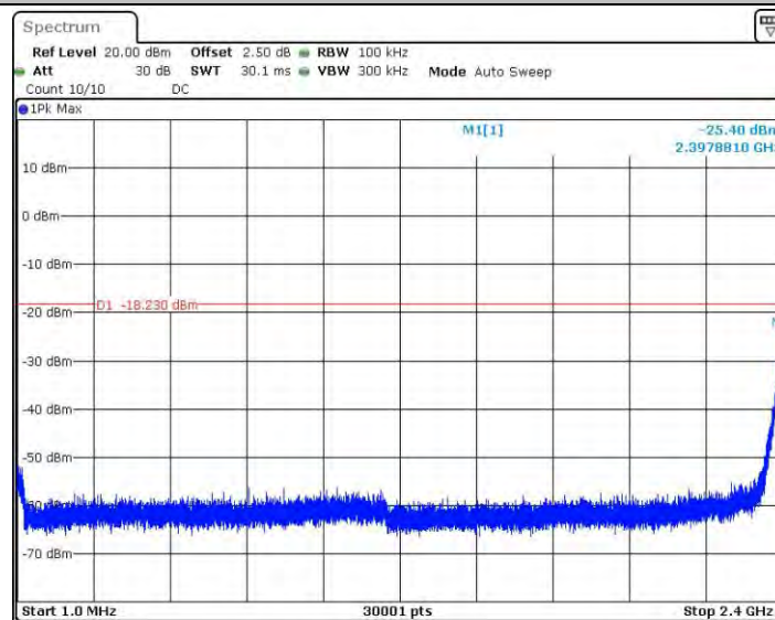
11N40_Ant2_2422_1~2400
