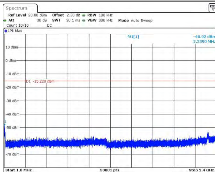
11N20_Ant1_2462_1~2400
