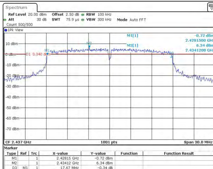
11N20_Ant2_2437
