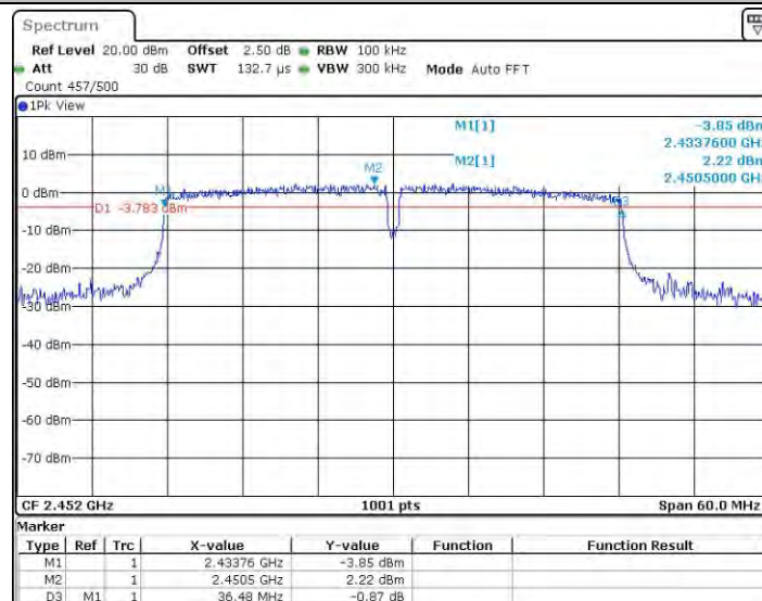
11N40_Ant2_2452
