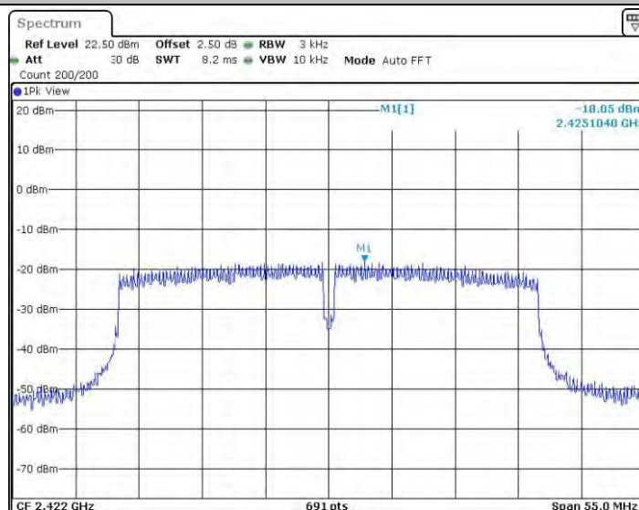
11N40_Ant2_2422
