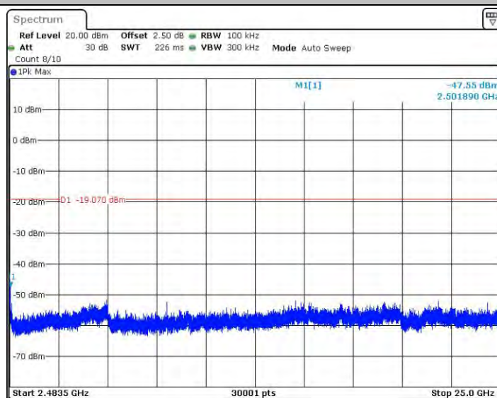
11N40_Ant1_2422_2483.5~25000
