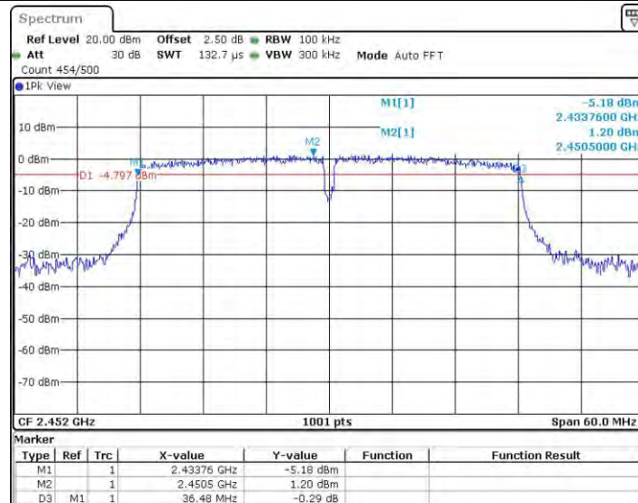
11N40_Ant1_2452
