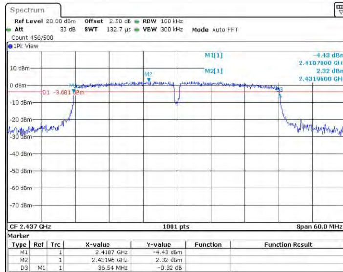
11N40_Ant2_2437
