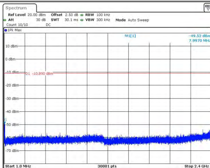
11B_Ant2_2462_1~2400
