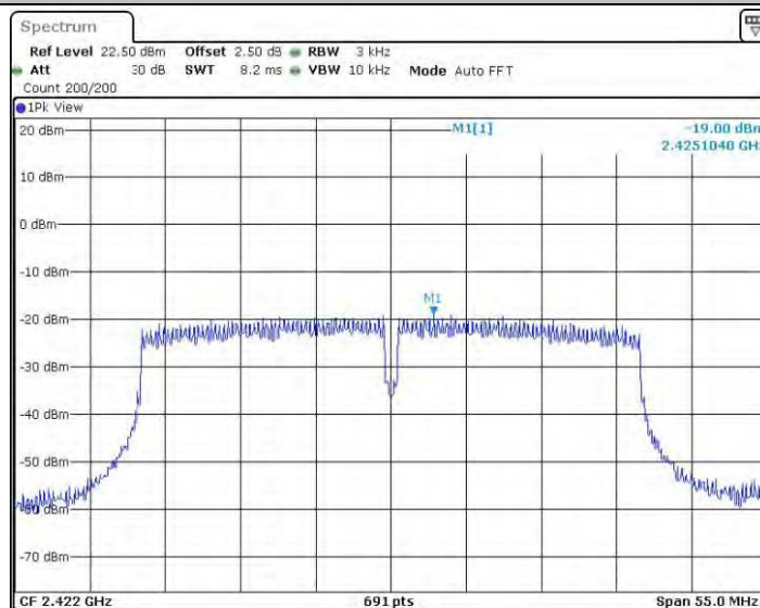
11N40_Ant1_2422
