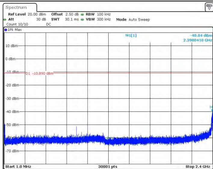
11B_Ant2_2412_1~2400
