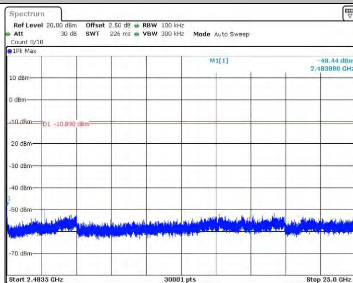
11B_Ant2_2462_2483.5~25000
