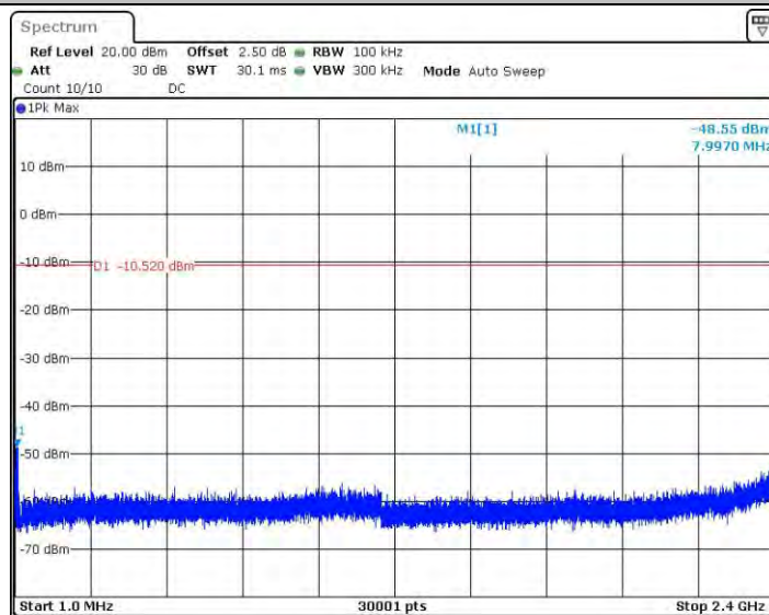
11B_Ant2_2437_1~2400
