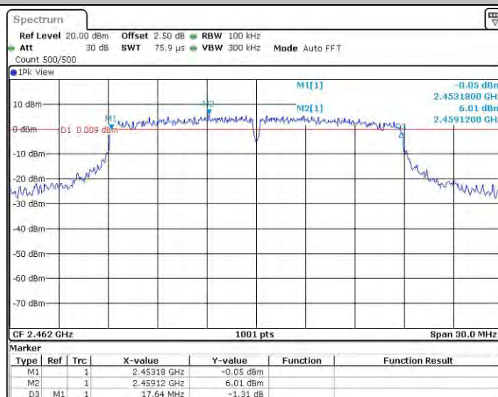
11N20_Ant1_2462
