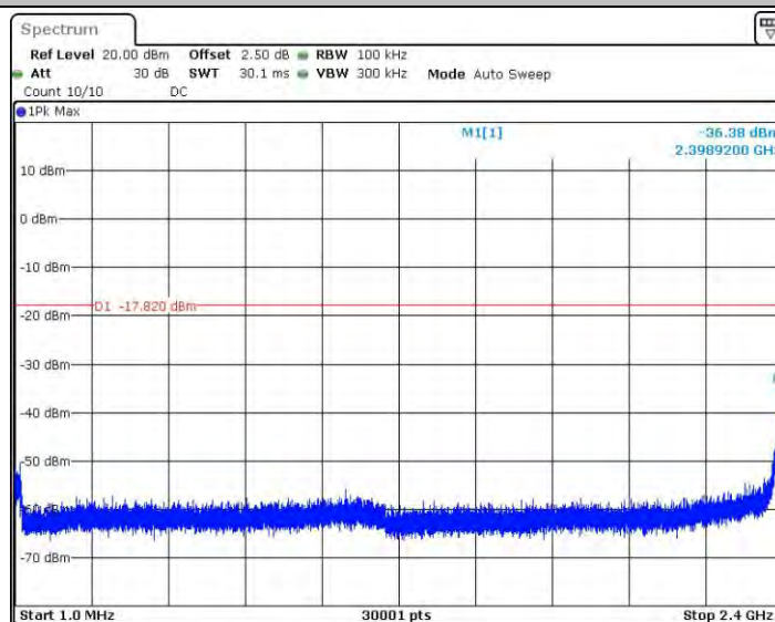
11N40_Ant2_2452_1~2400
