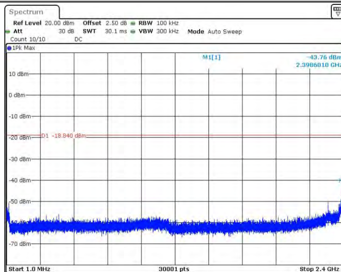
11N40_Ant1_2452_1~2400
