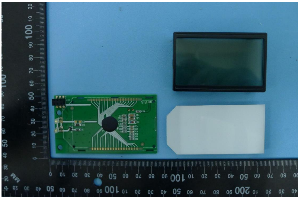
(12) EUT Photo
