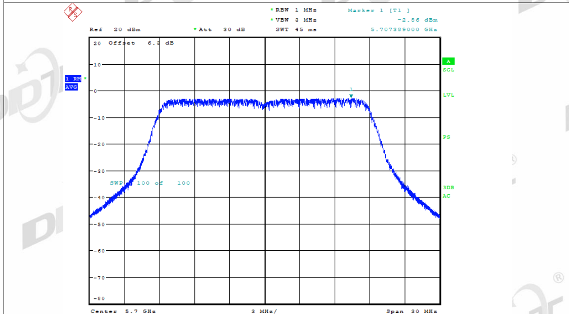
PSD NVNT ac20 5700MHz Ant2
