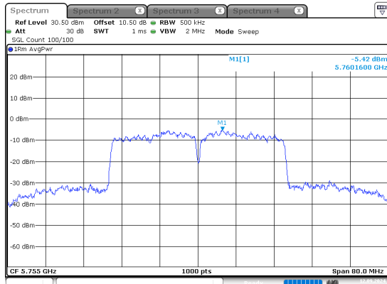
n40_5755MHz
