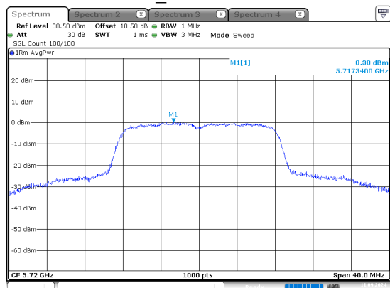
a_5720MHz
