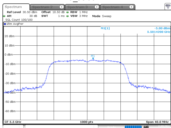
n20_5500MHz
