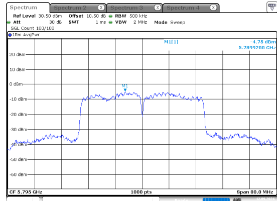
n40_5795MHz
