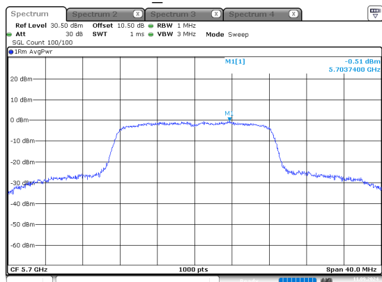
a_5700MHz
