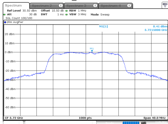
n20_5720MHz
