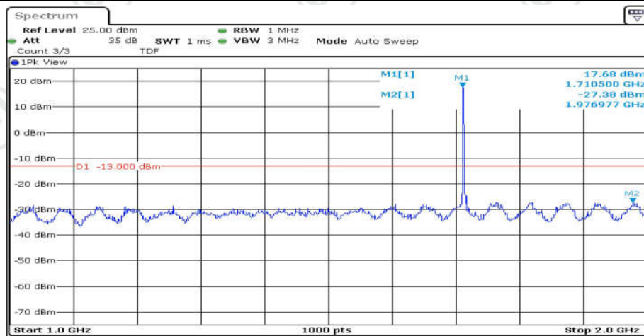
Band4-3MHz-16QAM-19965-1RB#0-Range2:1000~2000MHz
