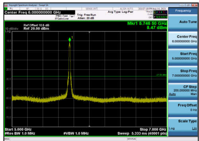
U-NII-3 ,Plot 3,5000MHz~7000MHz-802.1 1ac(20MHz),5745MHz,Ant1
