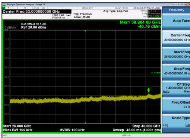
U-NII-3 ,Plot 2,26000MHz~40000MHz-802 .11ac(40MHz),5795MHz,Ant1
