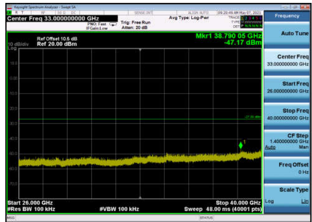
U-NII-3 ,Plot 2,26000MHz~40000MHz-802 .11ac(20MHz),5785MHz,Ant1
