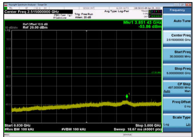
U-NII-3 ,Plot 2,30MHz~5000MHz-802.11a c(20MHz),5785MHz,Ant1
