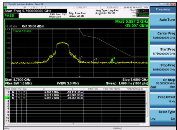
U-NII-3 ,Plot 1,Band Edge-802.11ac(40 MHz),5795MHz,Ant1
