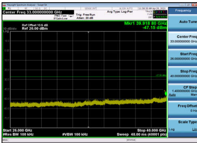
U-NII-3 ,Plot 2,26000MHz~40000MHz-802 .11ac(80MHz),5775MHz,Ant1
