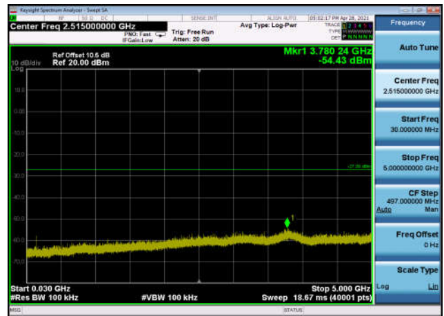
U-NII-3 ,Plot 2,30MHz~5000MHz-802.11a (20MHz),5825MHz,Ant1
