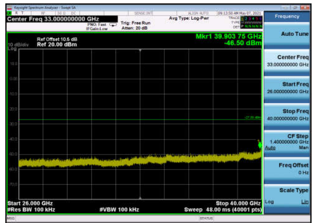
U-NII-3 ,Plot 2,26000MHz~40000MHz-802 .11ac(40MHz),5755MHz,Ant1
