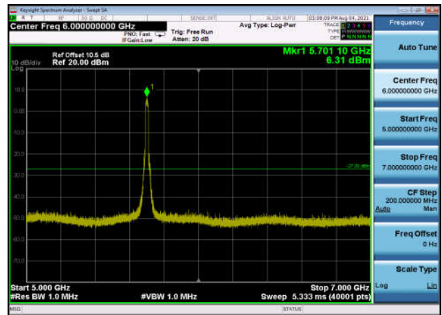
U-NII-2c ,Plot 3,5000MHz~7000MHz-802. 11ac(40MHz),5670MHz,Ant1
