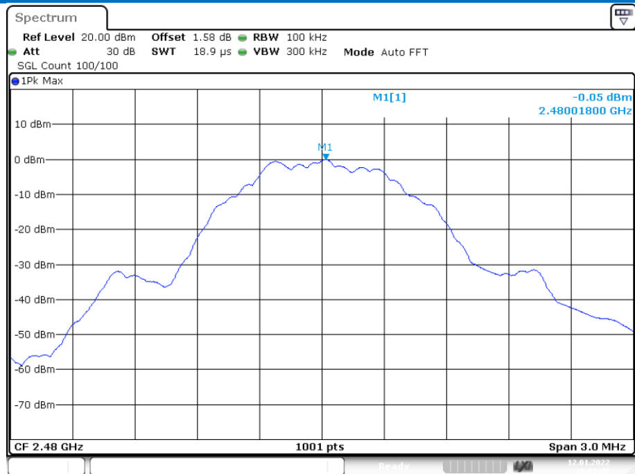
PSD NVNT BLE 1M 2480MHz
