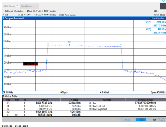
Band2-20MHz-QPSK-19100-100RB#0
