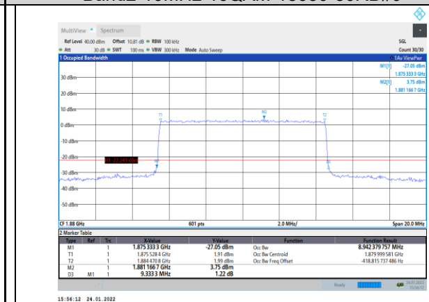
Band2-10MHz-16QAM-18900-50RB#0
