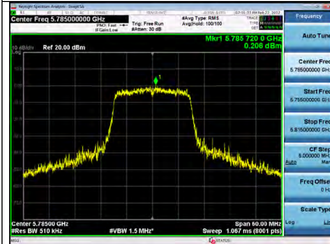
CH157 -5785MHz
