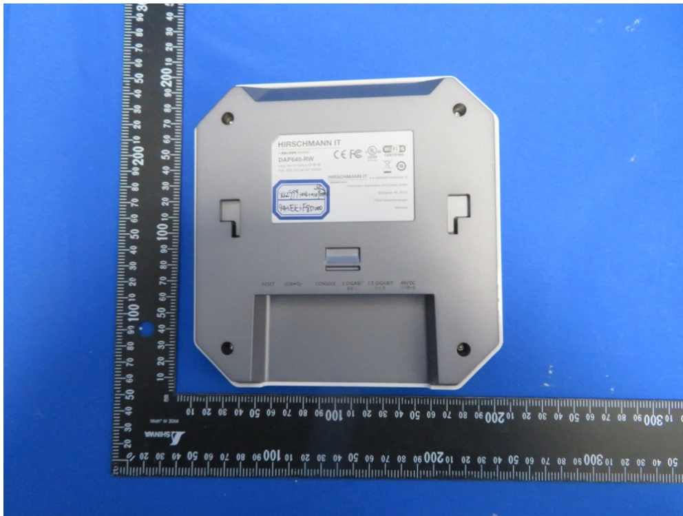
(5) EUT Photo (DAP640-RW)
