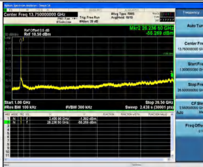
11N20_Ant2_2412_0~Reference
