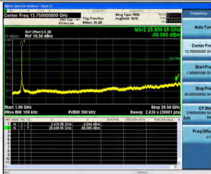
11N40_Ant2_2422_1000~26500
