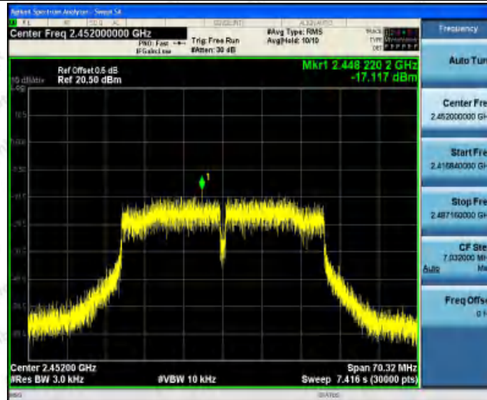
11N40_Ant2_2452
