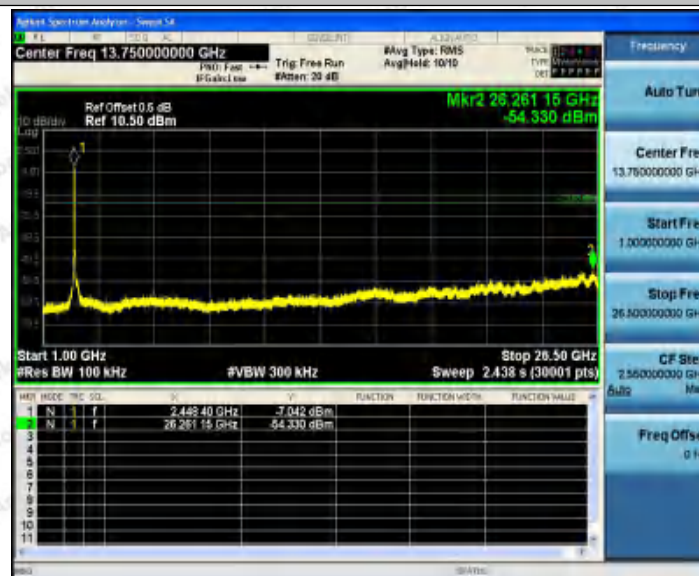
11N40_Ant2_2452_1000~26500
